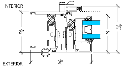
HINGED JAMB
