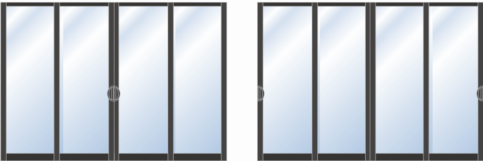
AL-PD OXXO
