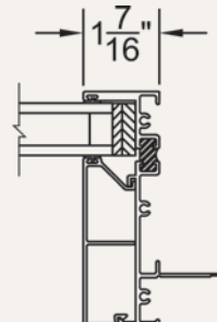
Jamb
