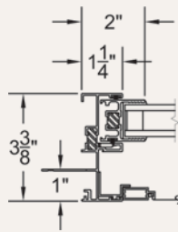
Lock Jamb
